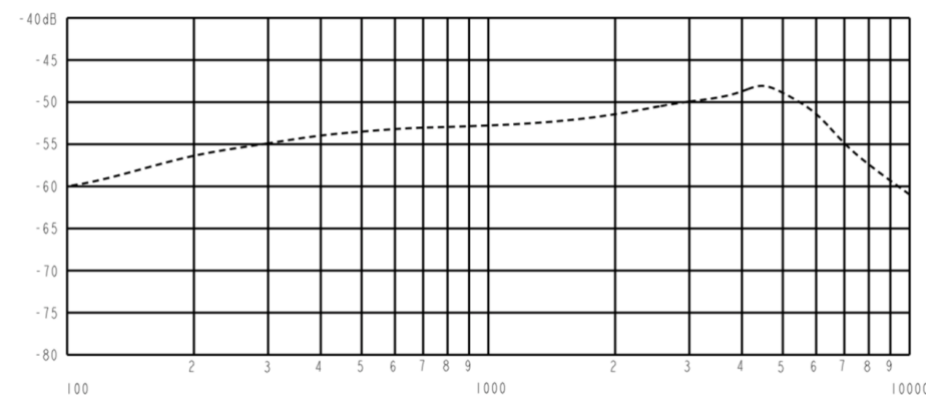
Рис.2 АЧХ МП-50У
