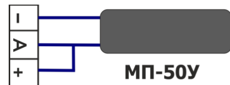
Рис.1 Схема подключения
